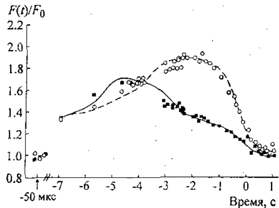
Рис. 5. Теоретические кривые получены для начальных условий, моделирующих воздействие наносекундного импульса высокой интенсивности (световая константа k_L = 6 \cdot 10^8 \text{ с}^{-1} ), включенного после измерительного света ( k_L = 0,6 \text{ с}^{-1} ). Расчет проведен для условий слабого измерительного света ( k_L = 0,6 \text{ с}^{-1} ) и параметров модели, описывающих нативный образец (сплошная линия) и образец в среде с диуроном (пунктирная линия). Результаты расчета сравниваются с экспериментальными данными для нативного (черные квадраты) образца и образца в среде с диуроном (светлые кружки).
